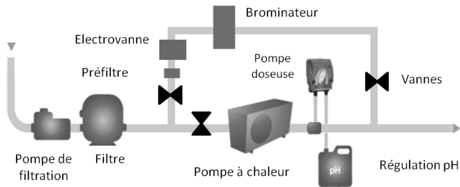
Figure 27. 1 ère possibilité d'installation du kit « régulation brome »
