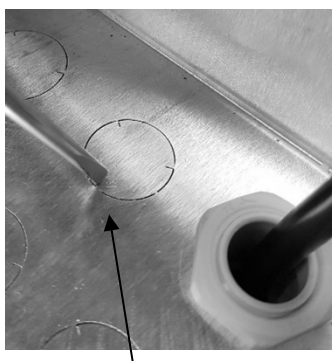
Figure 33. Ouverture et fixation du boîtier Kompact mini M9
