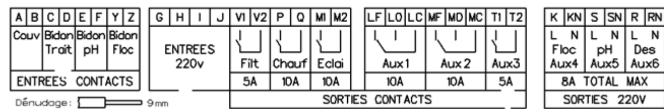
Figure 38. Entrées sorties de la centrale Kompact mini M9
