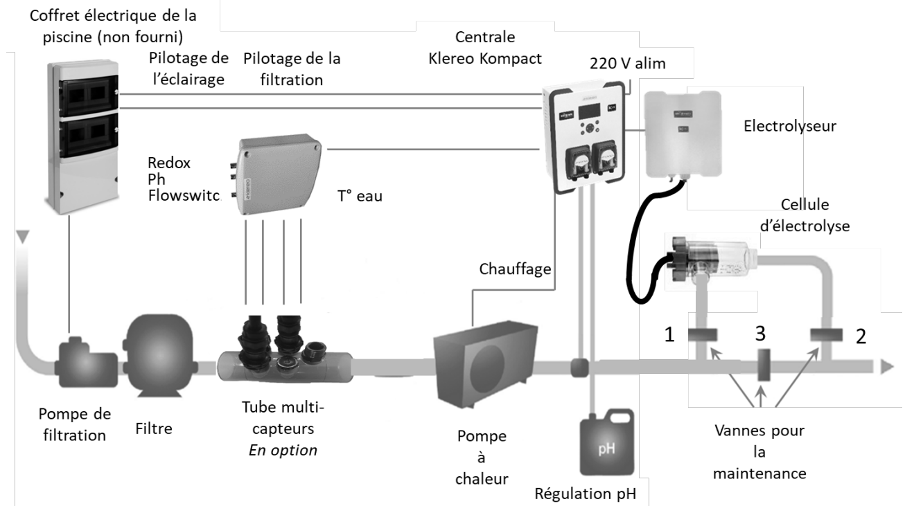
Figure 29. Installation de la cellule d'électrolyse
