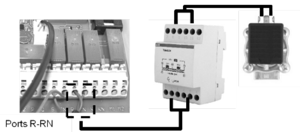
Figure 45. Branchement de l'électrovanne
