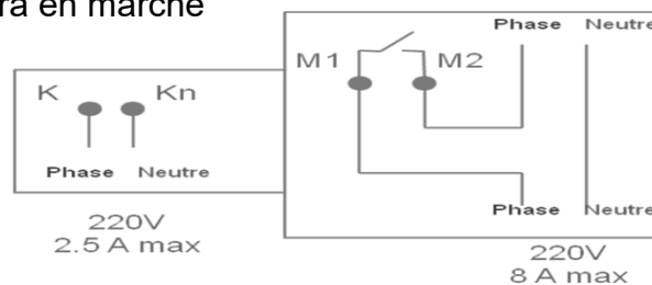
Figure 41. Câblage de la sortie double relais
