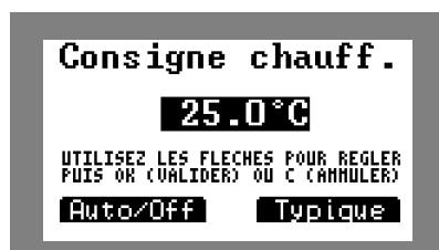
Figure 13. Ecran de réglage de la consigne chauffage
